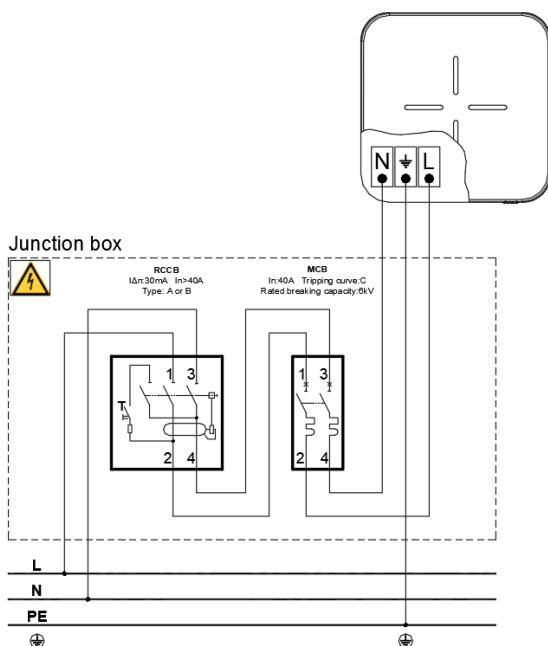
Fig. 14 Schema de cablaj a încărcătorului 1P7K*
